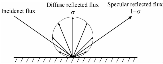
图 7 Maxwell 模型的示意图 Fig. 7 Sketch of the Maxwell model
