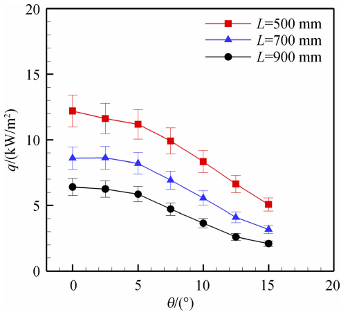
图 3 热流测量曲线
