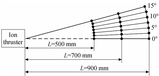
图 2 热流传感器测点分布
