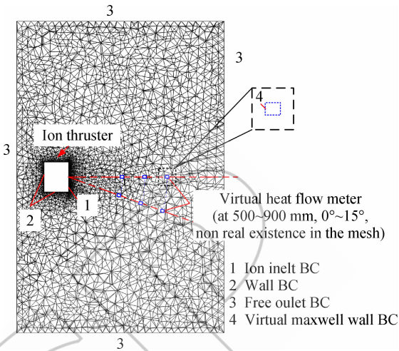
图 5 仿真中使用的网格 2D-cutplan
