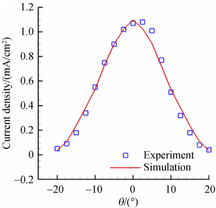
图 4 EX-PWS 计算得到的 500 mm 处束电流密度和实验结果的对比
