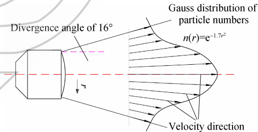
图 6 离子推力出口分布条件 [12]
